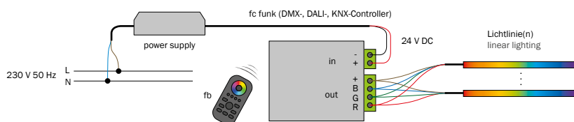
Anschlussplan RGB mit Funk, casambi, DMX, KNX • Wiring diagram for RGB with wireless, Casambi, DMX and KNX
