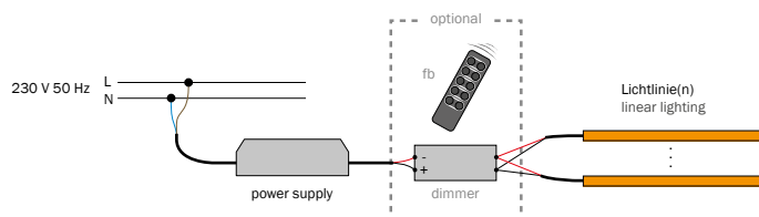
Anschlussplan einfarbige Lichtlinie ohne dimmer • Wiring diagram for a single-colour light strip without a dimmer
